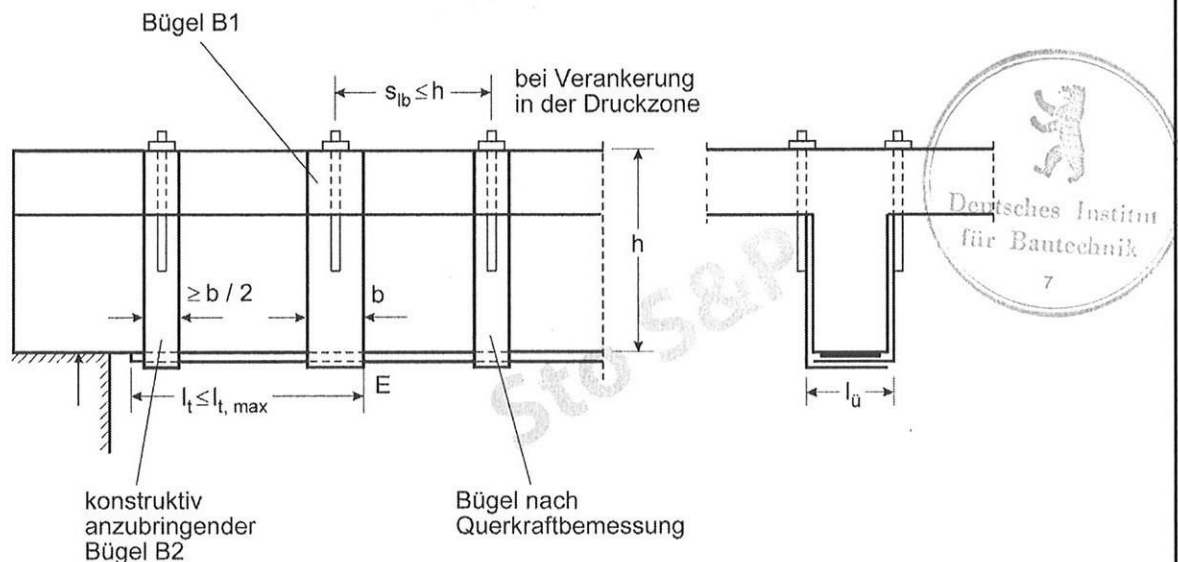
Bild 4: Verbügelung der Lamellenverankerung (Beispiel für Bügelverankerung in der Druckzone)
