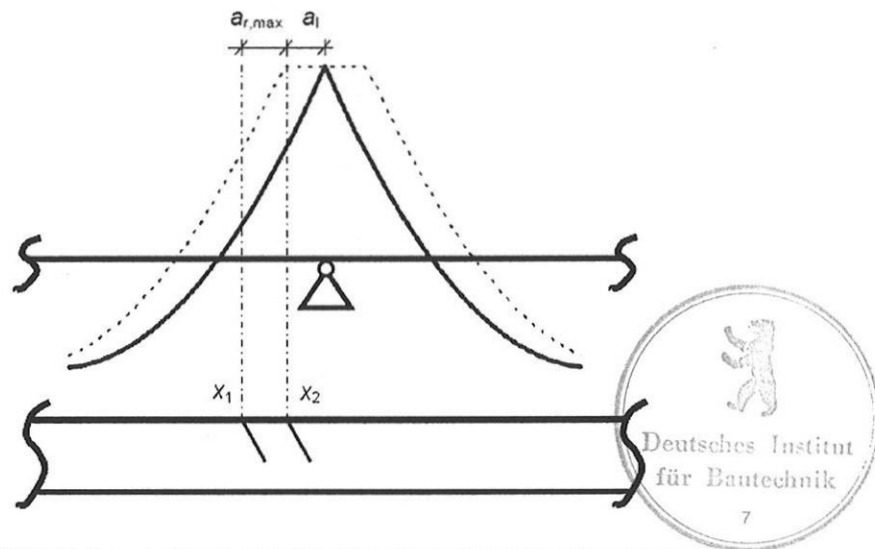
Bild 5: Lage des betrachteten Zwischenrisselements
