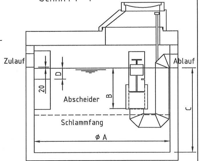
Schnitt I - I
