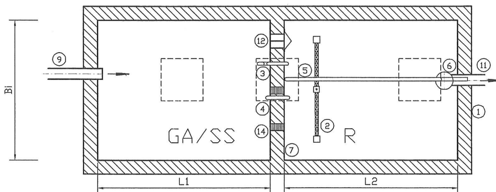
Draufsicht
