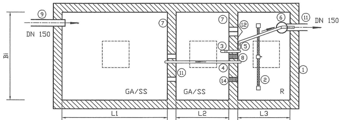
Draufsicht
