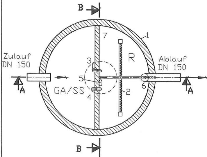
Draufsicht
