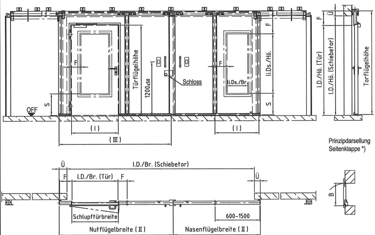
T90-2 Prinzipdarstellung *)
