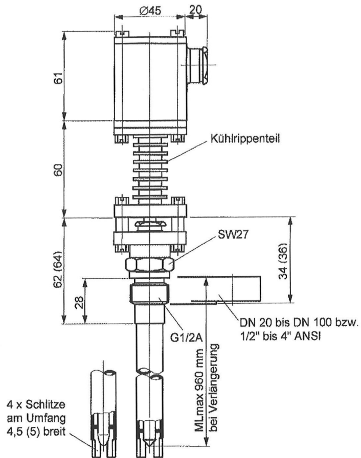
Schema der Überfüllsicherung
