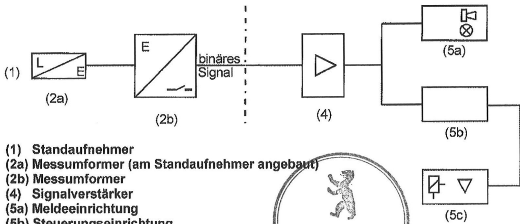
Schema der Überfüllsicherung
