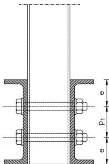
Schnitt A-A
