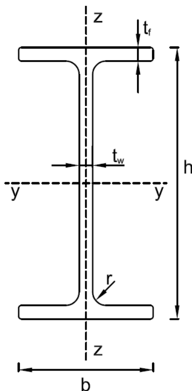
Bild A-1: Doppel-T-Profil
