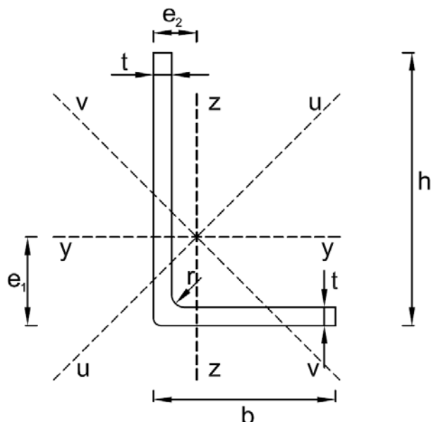
Bild A-3: Winkelprofil
