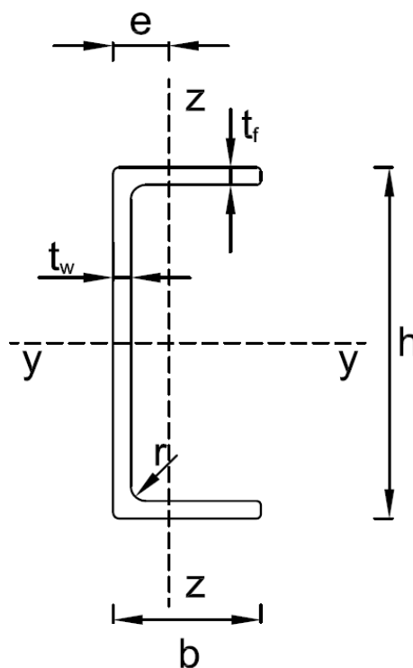
Bild A-2: U-Profil
