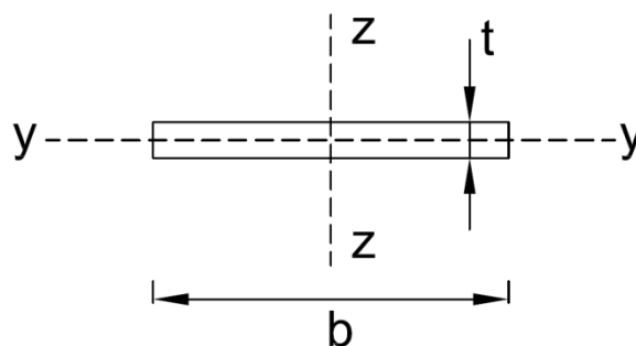
Bild A-5: Flachprofil
