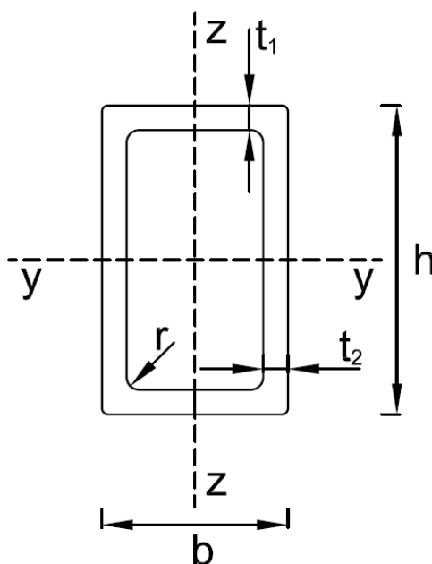
Bild A-4: Vierkanthohlprofil
