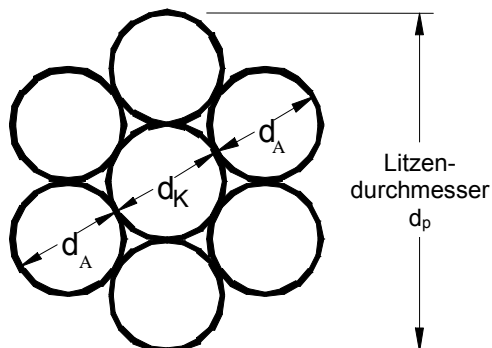
Bild 1: Litzenquerschnitt
