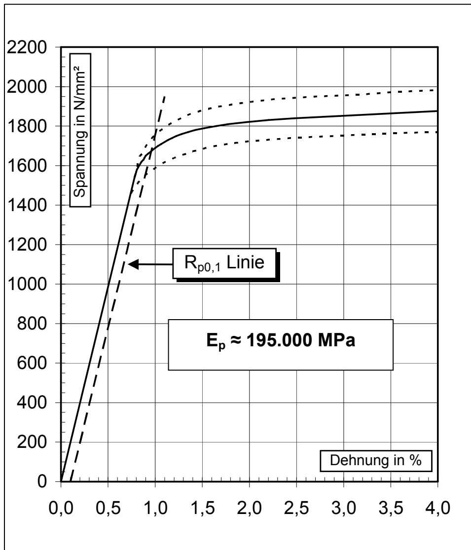
Bild 2: Spannungs - Dehnungslinie
