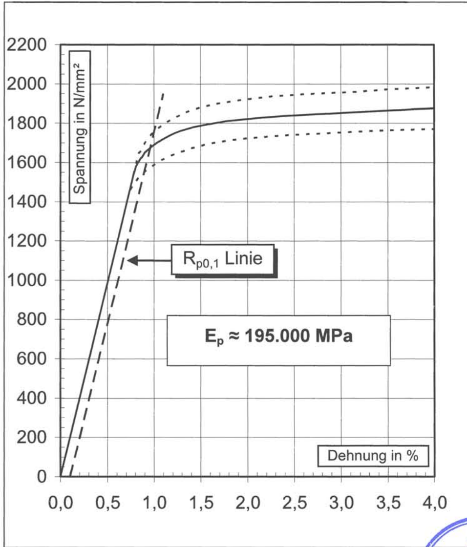
Bild 2: Spannungs – Dehnungslinie
