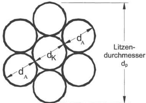
Bild 1: Litzenquerschnitt
