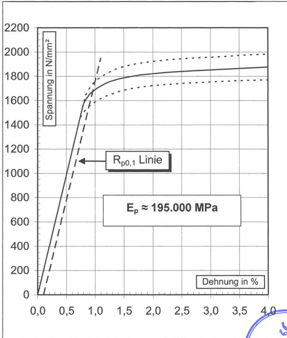
Bild 2: Spannungs - Dehnungslinie
