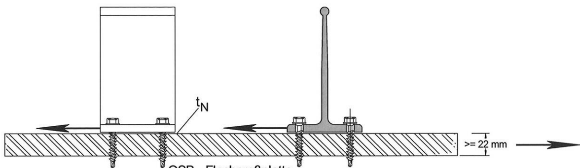
OSB - Flachpreßplatte
