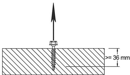
Vollholz S10 / C24
