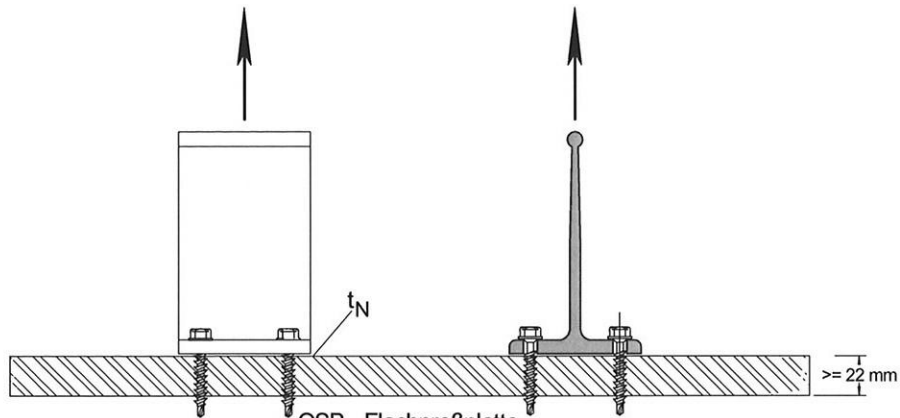
OSB - Flachpreßplatte
