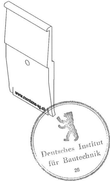
MONTAFIX®-Halter
