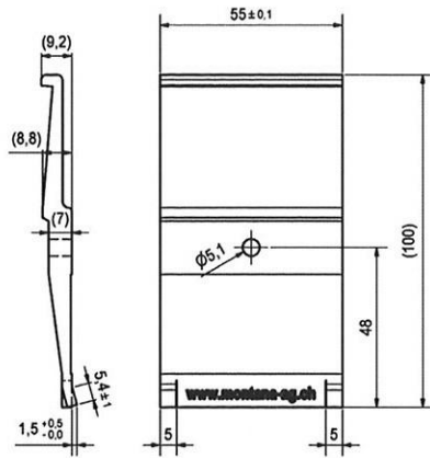
MONTAFIX®-Halter
