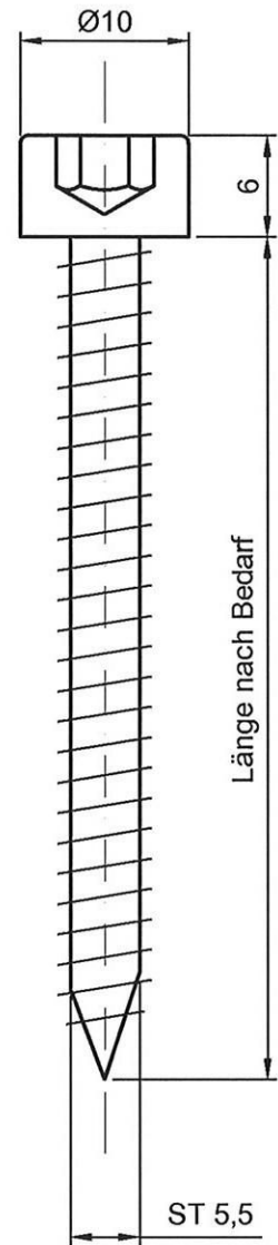
Blechschaube mit Innensechskant ST5,5x38, A4 Kopf nach DIN 912
