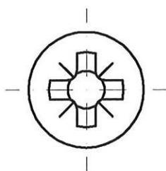
Linsensenk-Blechschaube ST5,5x60-C-Z A2, ISO 7051 Sternantrieb T20/T25 oder Kreuzschlitz
