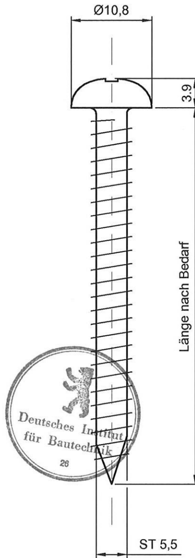
Linsenkopf-Blechschaube ST5,5x50, A4, ISO 7049 Sternantrieb T20/T25 oder Kreuzschlitz
