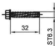
gewindefurchende Blechschaube ST6.3x32 (A4-70)
