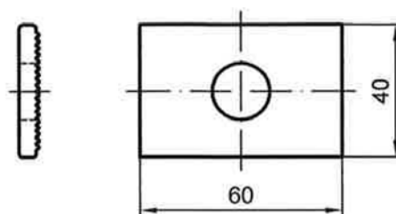
Unterlegplatte (266977 FZ 0300)
