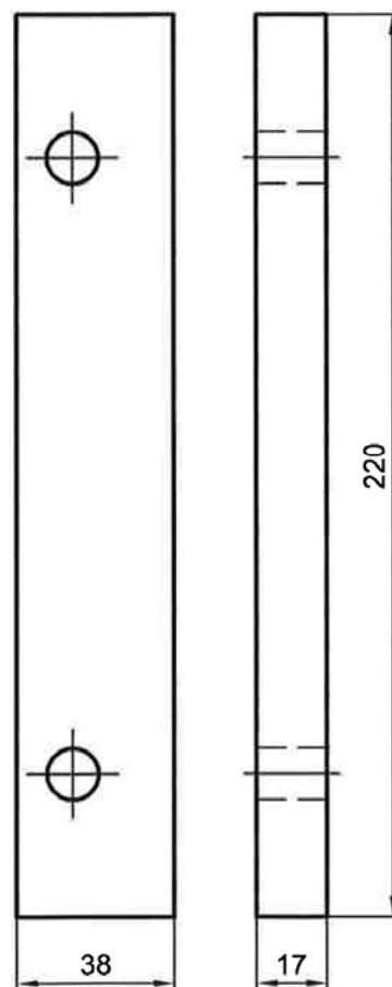
Füllstück (267895 FZ 0100)
