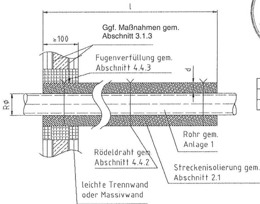
Schnitt – Einzeldurchführung
