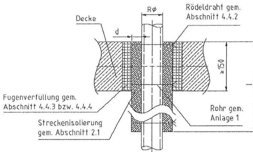
Schnitt – Einzeldurchführung
