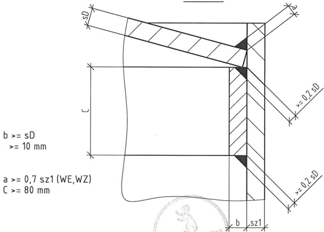
Einzelheit Z
