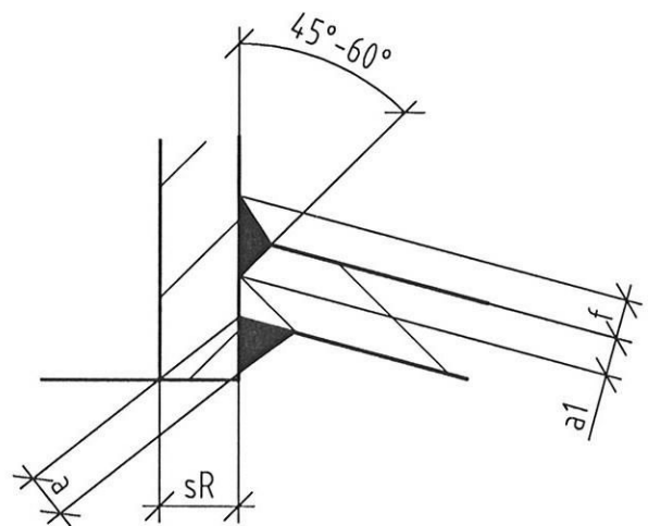
Einzelheit Z
