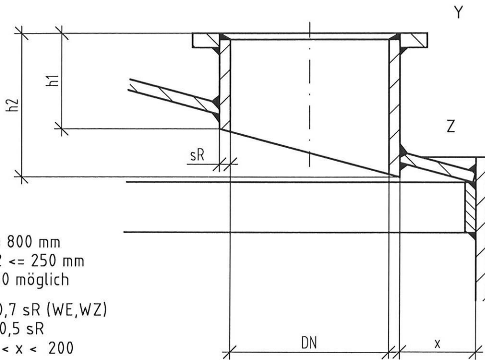
Einzelheit Y
