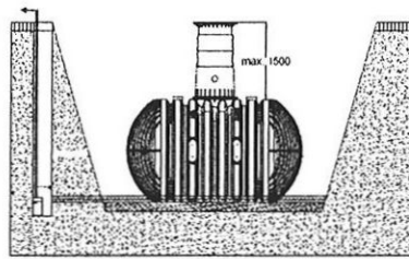
Überdeckungshöhen mit Zwischenstück und Teleskop Domschacht maximal (nur im Grünbereich ohne Grund- und Schichtenwasser). Eine Drainage wird generell empfohlen.
