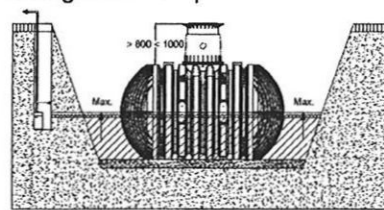
Überdeckungshöhen bei Installation in Grundwasser – die schraffierten Flächen geben die zulässige Eintauchtiefe für die daneben stehende Tankgröße an (nicht unter PKW oder LKW befahrenen Flächen)
