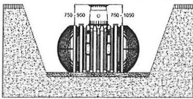
Überdeckungshöhen mit Teleskop Domschacht im Grünbereich
