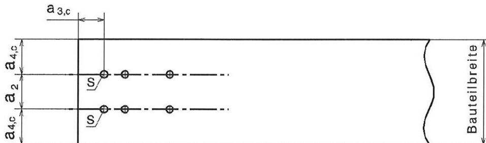
Draufsicht
