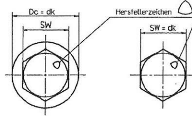
Außensechskant mit Flansch
