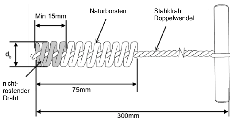
Doppelfaserbürste Durchmesser d_b entsprechend Tabelle 4
