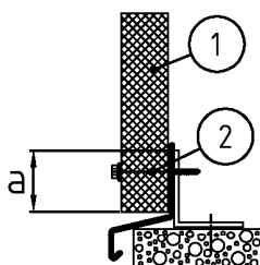
Bild 4 : Fußpunkt Wandpaneel
