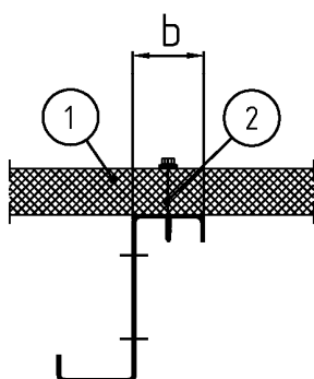
Bild 1 : Stahlaufleger
