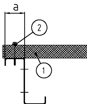
Bild 4 : Traufpunkt
