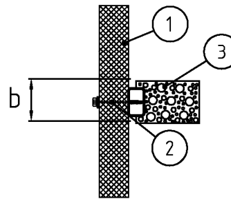
Bild 3 : Betonaufleger
