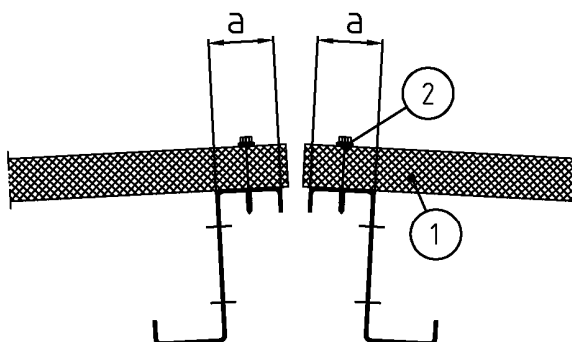
Bild 5 : First
