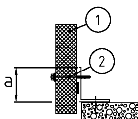
Bild 5 : Fußpunkt Wandpaneel- Vorgesetzt
