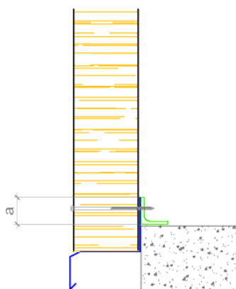
Bild 5 Fusspunkt Wandelement vorgesetzt
