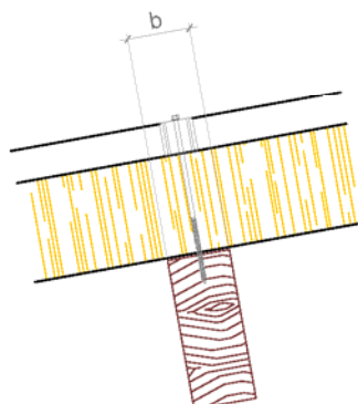
Bild 2 Holzaufleger
