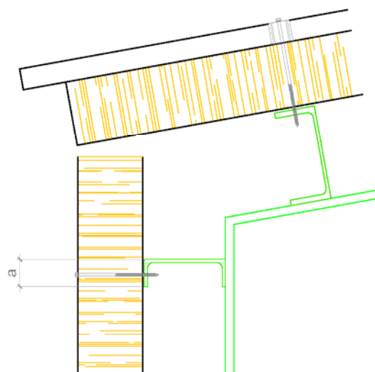
Bild 6 Traufpunkt
