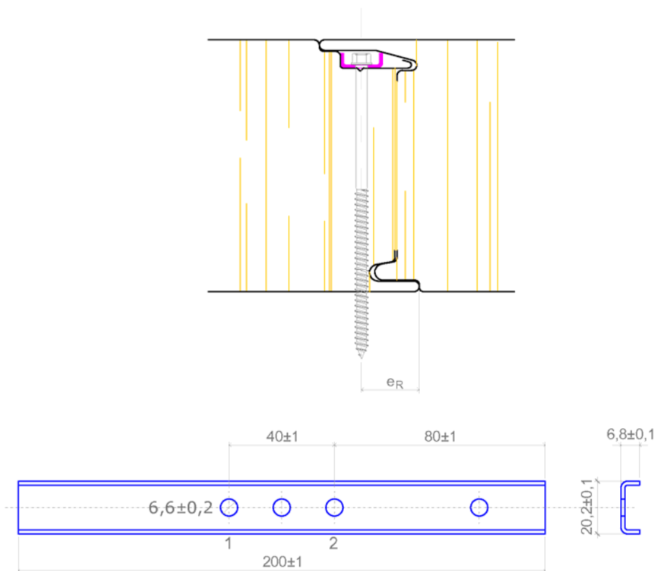
Lastverteilerplatte aus verzinktem Stahl DX51 ( t = 1,5 \pm 0,1 mm)
