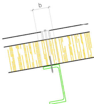
Bild 1 Stahlaufleger
