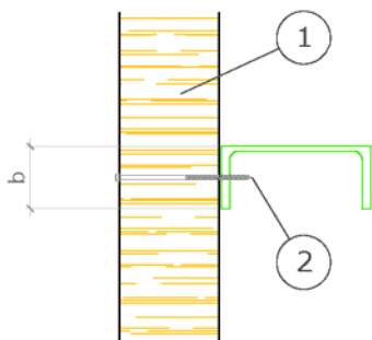
Bild 1 Stahlaufleger
