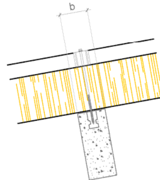
Bild 3 Betonaufleger
