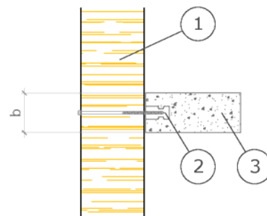
Bild 3 Betonaufleger
