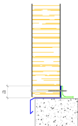
Bild 4 Fusspunkt Wandelement aufgesetzt
