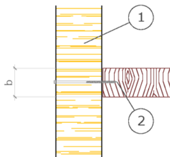
Bild 2 Holzaufleger
