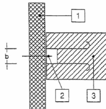
Bild 3 Betonaufleger
