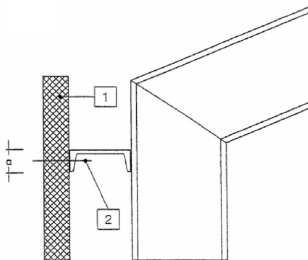
Bild 6 Traufpunkt
