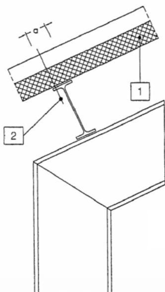
Bild 4 Traufpunkt
