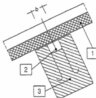
Bild 3 Betonaufleger
