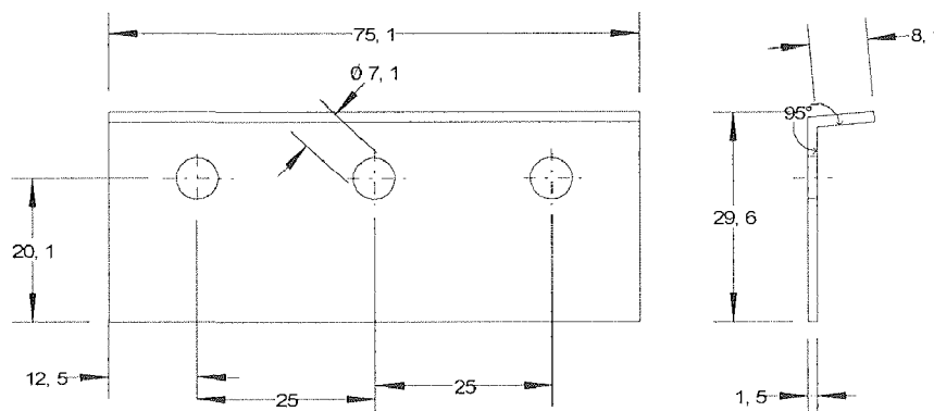
Lastverteilerschiene (Werkstoffnummer 1.4301)
