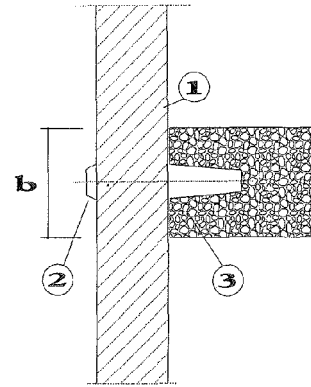
Bild 3 Betonaufleger
