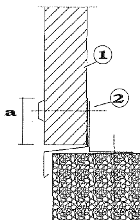
Bild 5 Fußpunkt Wandelement vorgesetzt
