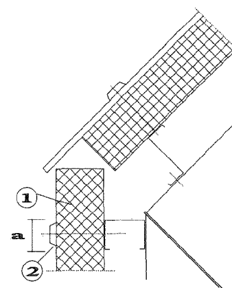
Bild 6 Traufpunkt
