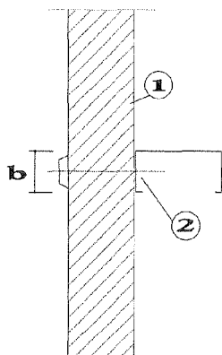
Bild 1 Stahlaufleger
