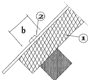
Bild 2 Holzaufleger
