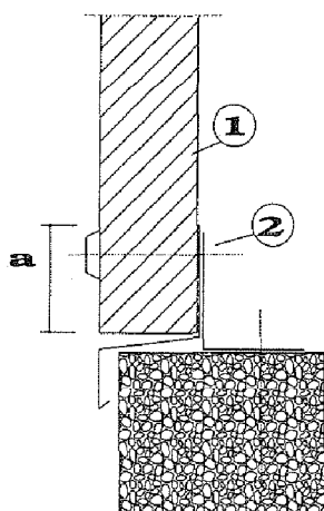
Bild 4 Fußpunkt Wandelement aufgesetzt
