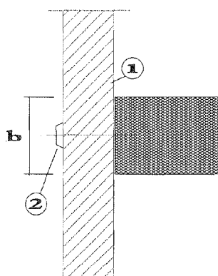
Bild 2 Holzaufleger
