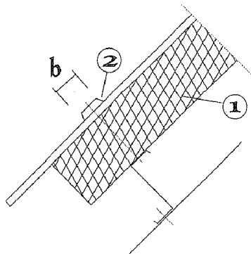
Bild 1 Stahlaufleger
