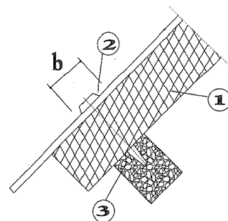
Bild 3 Betonaufleger
