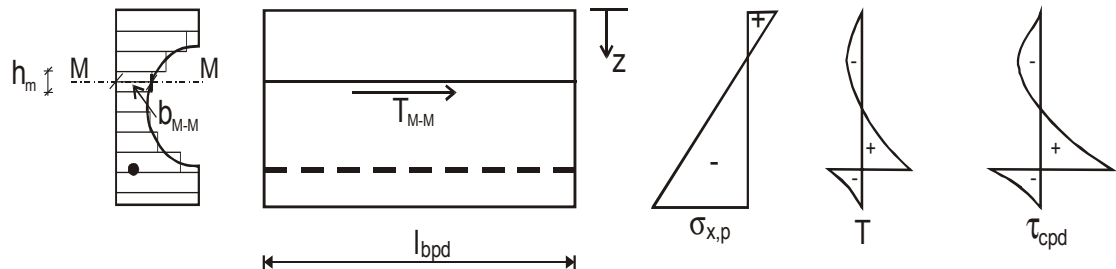
Bild 1: Ermittlung der Schubspannung aus Spannkrafteinleitung
