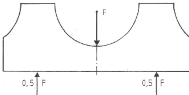
Bild 1: Belastungsanordnung Biegeversuch
