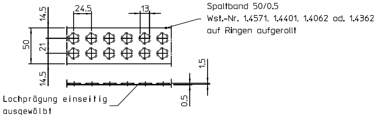
MOSO - Wellbügel: Wst.-Nr. 1.4571, 1.4401, 1.4062 oder 1.4362
