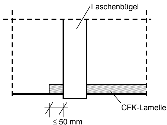
Bild 3: Anordnung des Stahllaschenbügels am Lamellenende
