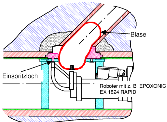
Bild 7: Schritt 6 Verpressen des EPOXONIC- Materials
