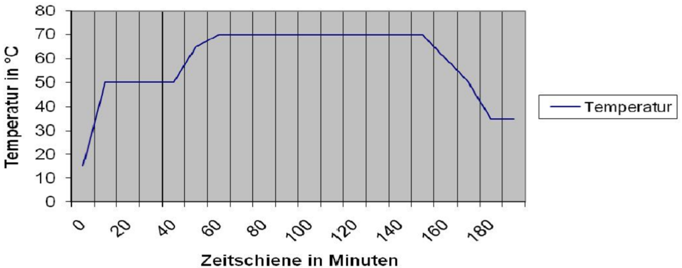
Heizkurve FluviPox TF 8 bei Dampfaushärtung
