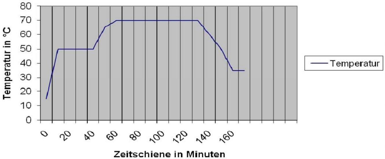
Heizkurve FluviPox TF 4 bei Dampfaushärtung
