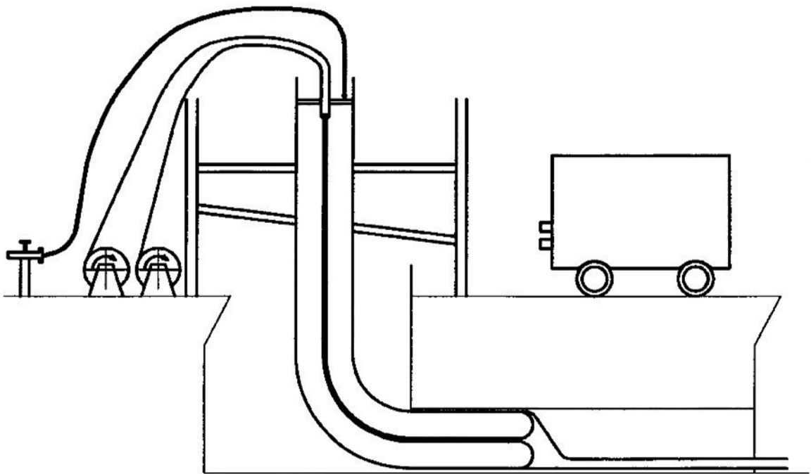
Der Kalibrierschlauch inversiert in den bereits positionierten Schlauchliner
