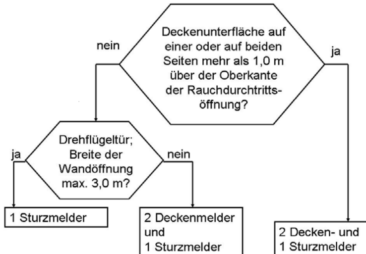
Bild 3: Entscheidungsdiagramm
