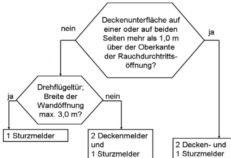
Bild 3: Entscheidungsdiagramm
