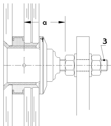
a) maßgebende Länge für Bolzenauswahl 3) Bolzenauswahl nach Tabelle
