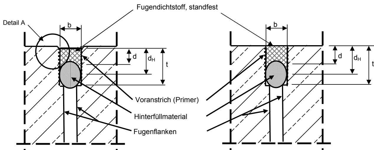
Befahrbare Fugenkonstruktion
