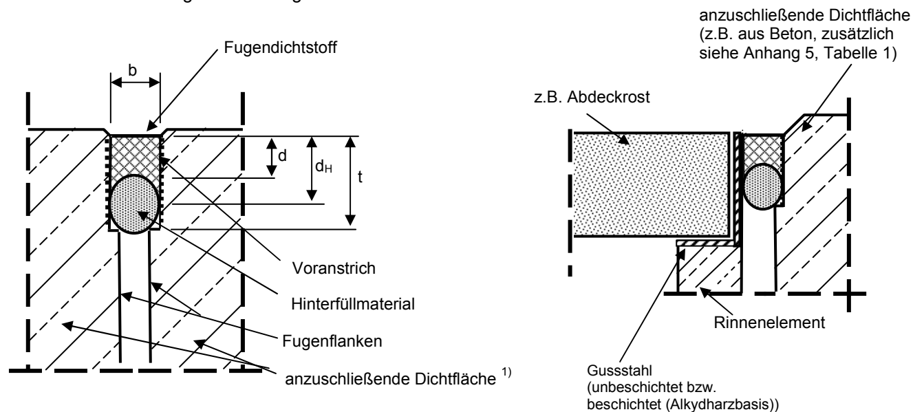
Bild 1: befahrbare Fugenausbildung
