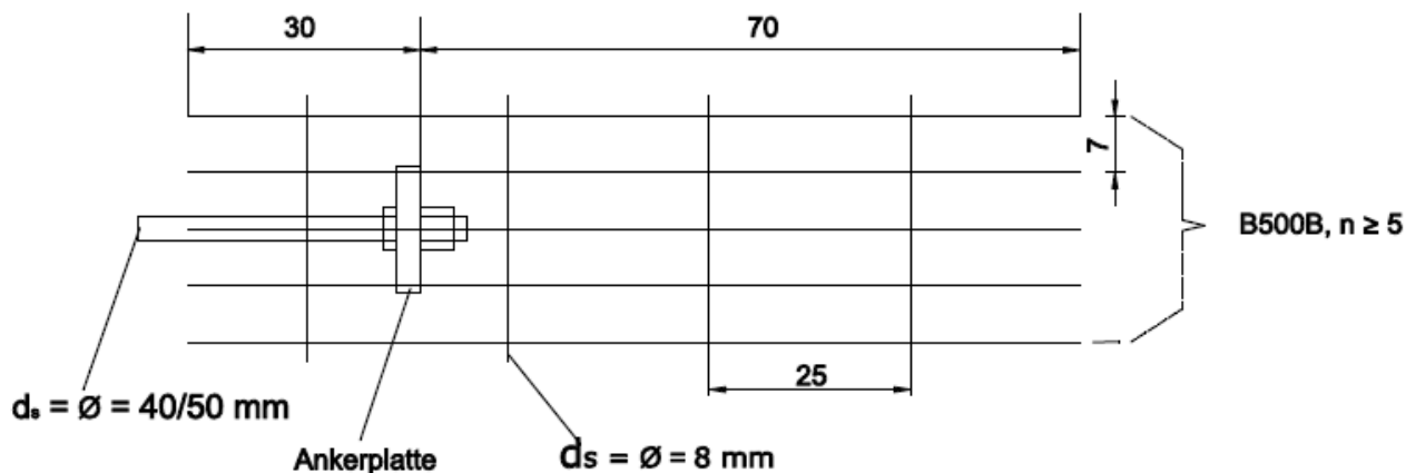
Bild 5: Beispiel für die Bewehrung einer Stütze
