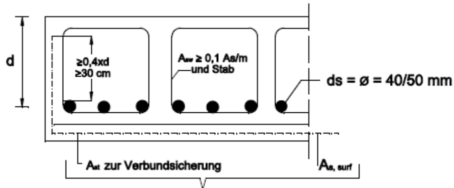
Bild 4a: Platten mit und ohne rechnerisch erforderliche Querkraftbewehrung
