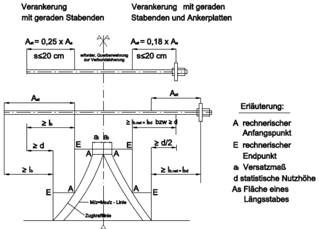
Bild 3b: Beispiel für die Verankerung von Stäben d_s bzw. \Phi = 40 und 50 mm mit geraden Stabenden und Ankerplatten im Stützbereich massiger Bauteile nach Abschnitt 4.3.2
