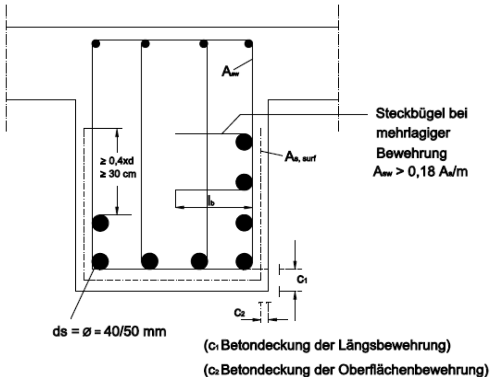
Bild 4b: Balken und Anordnung von Steckbügeln bei mehrlagiger Bewehrung
