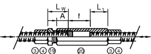
Bild 10 Muffenstoß - Spannschloß Ø40 - 50
