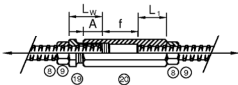
Bild 5 Muffenstoß - Spannschloß Ø40 - 50
