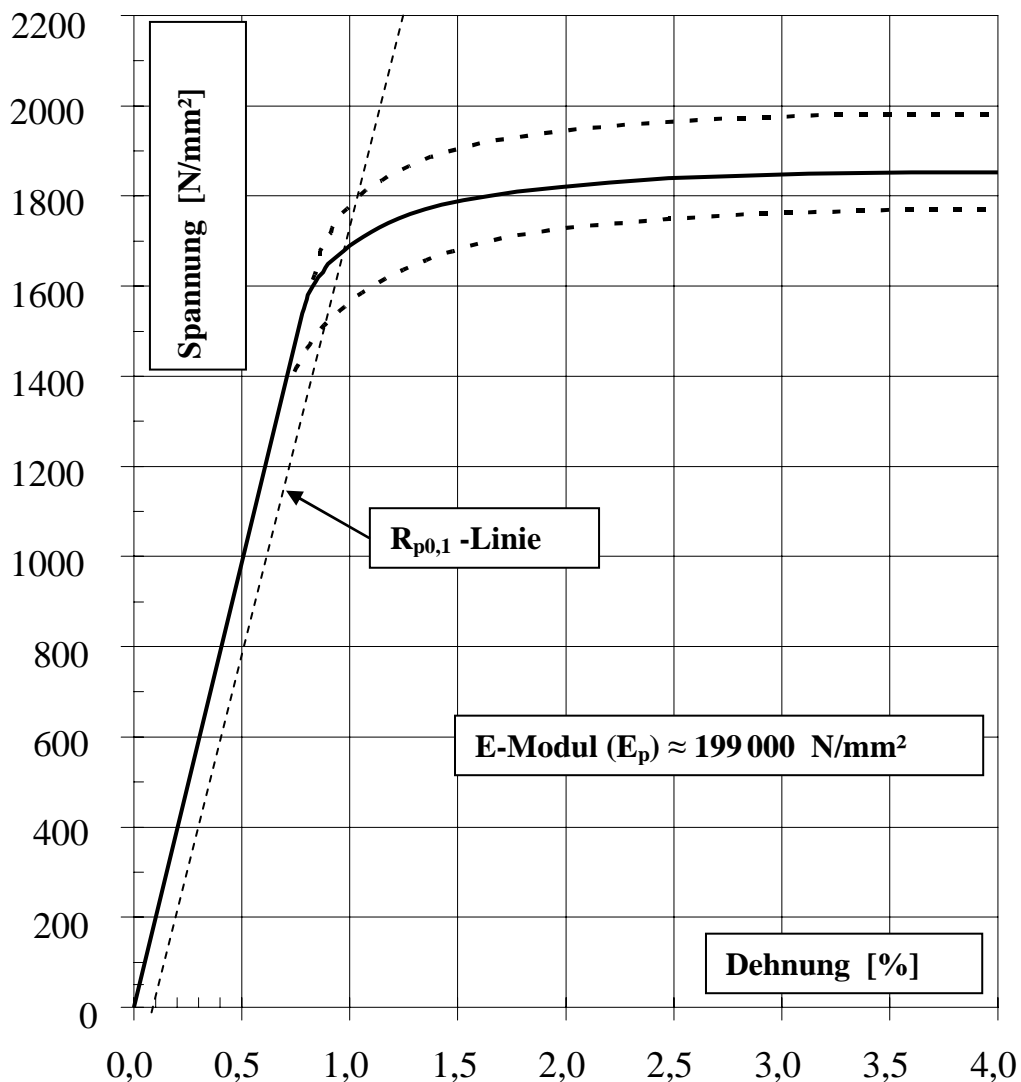
Bild 2 : Spannungs - Dehnungslinie
