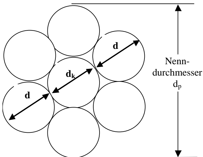
Bild 1: Litzenquerschnitt
