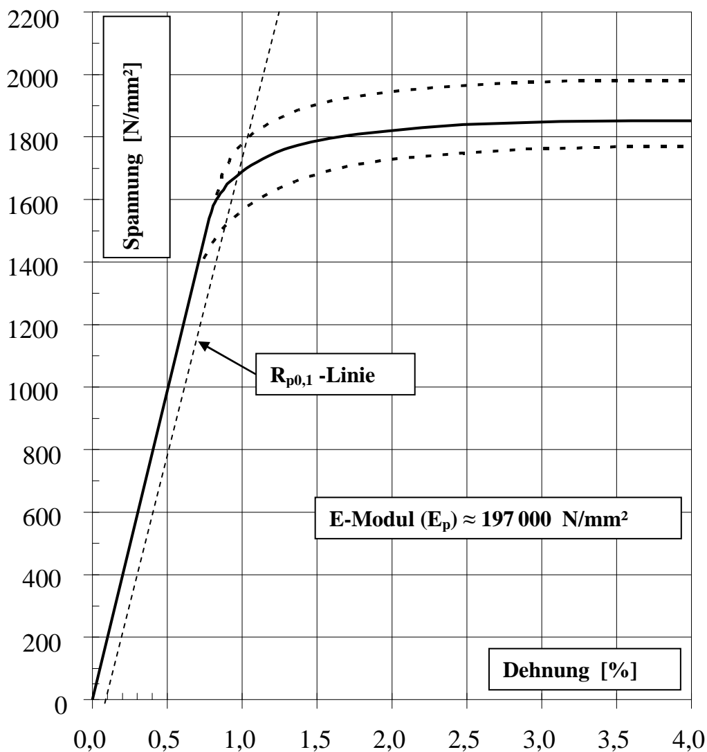
Bild 2: Spannungs - Dehnungslinie
