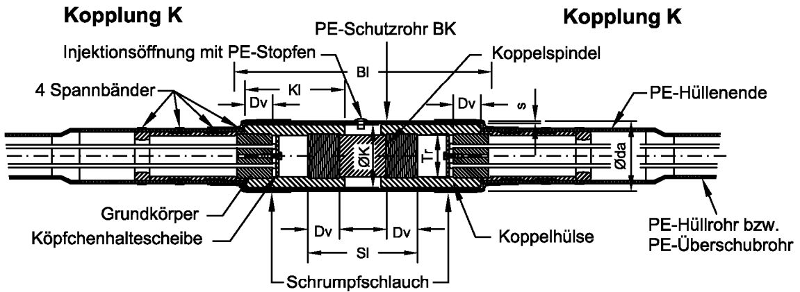
Feste und bewegliche Kopplung
