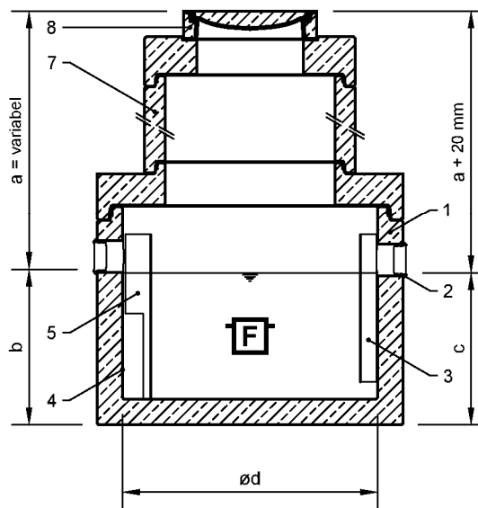
Maße Fettabscheider
