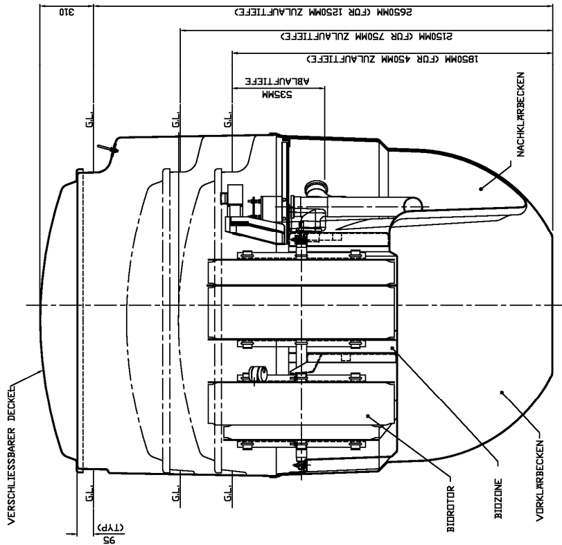
DECKEL, BIODISCD, SEITENANSICHT
