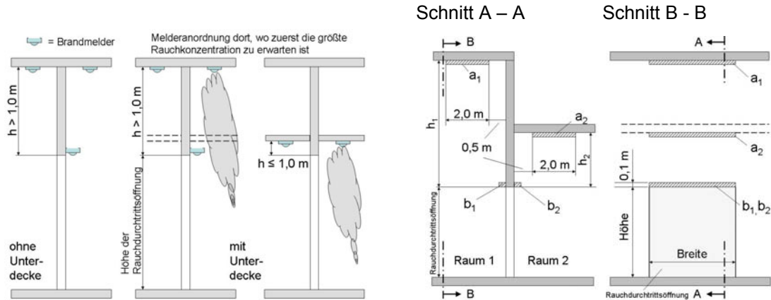
Bild 1: Maßgebende Höhe der Deckenunterfläche Bild 2: Installationsbereiche
