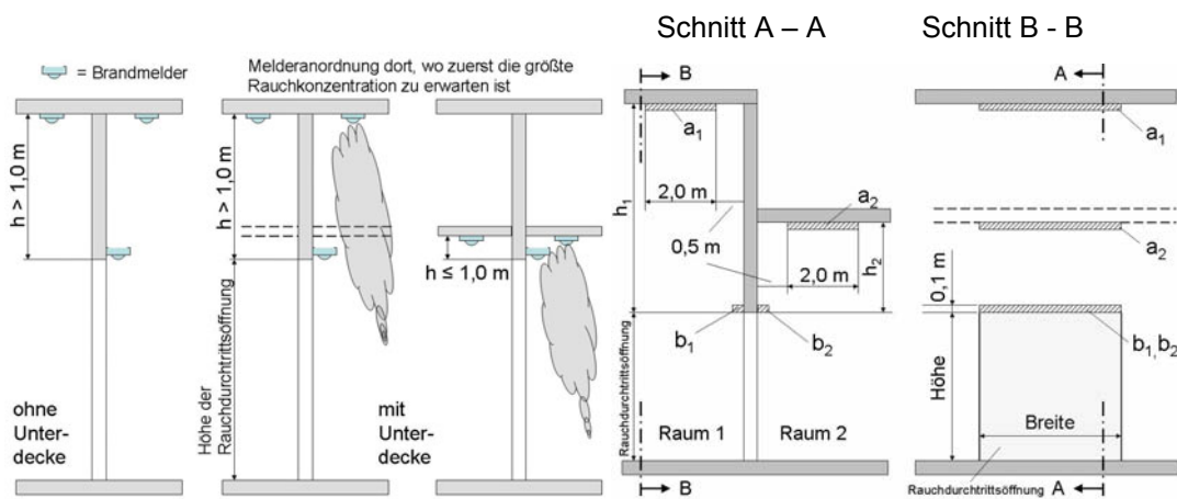
Bild 1: Maßgebende Höhe der Deckenunterfläche
