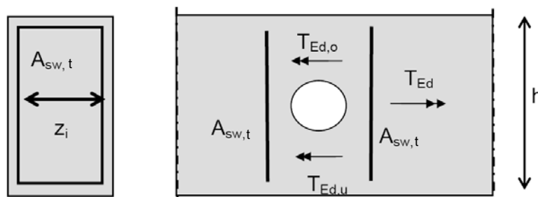
Bild 4: Innerer Hebelarm z_i und Anordnung der Bügelbewehrung A_{sw,t} vor und hinter jeder Öffnung bei kippsgefährdeten Trägern
