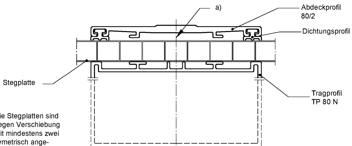
Schnitt C-C
