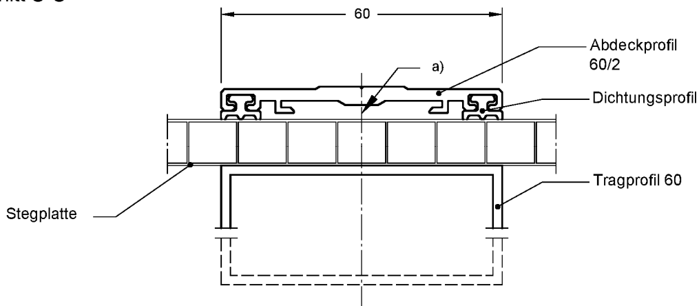
Schnitt C-C
