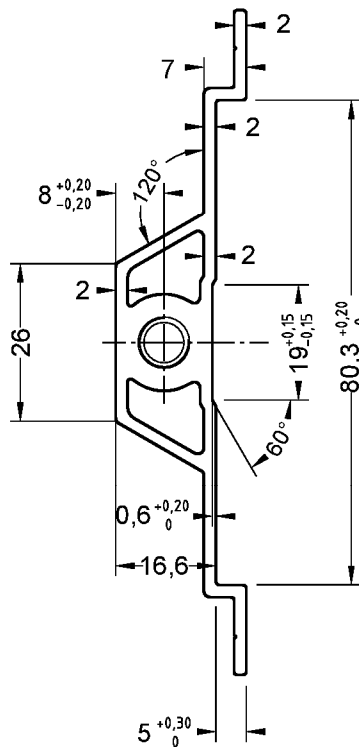
Spannschloss, Unterteil 80
