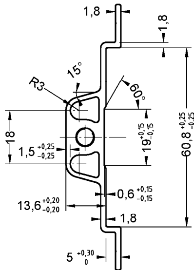
Spannschloss, Unterteil 60
