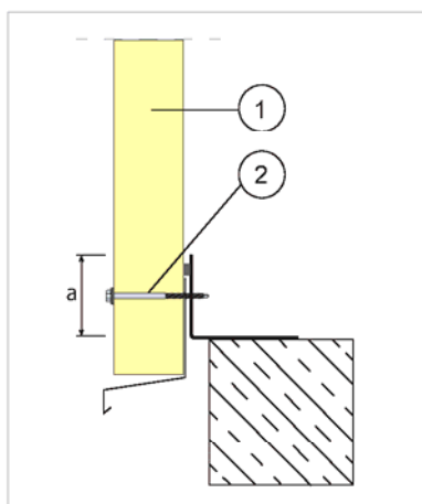
Bild 4: Fußpunkt Wandpaneel - aufgesetzt
