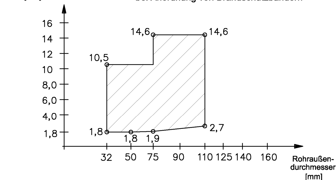
Rohre gemäß Rohrgruppe B-2 der Anlage 1 für Einbau der Kombiabschottung in Decken (Ausführungsvariante 2) bei Anordnung von Brandschutzbändern
