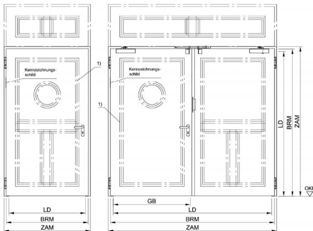
Dargestellt: Gangflügel DIN links, Gangflügel DIN rechts spiegelbildlich
