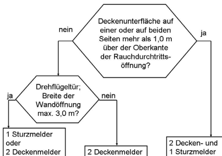
Bild 3: Entscheidungsdiagramm
