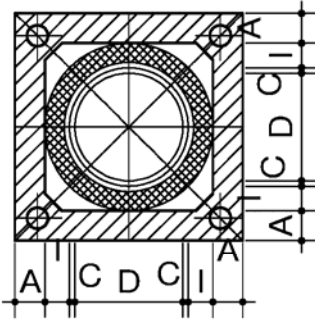
Einzelschornstein
