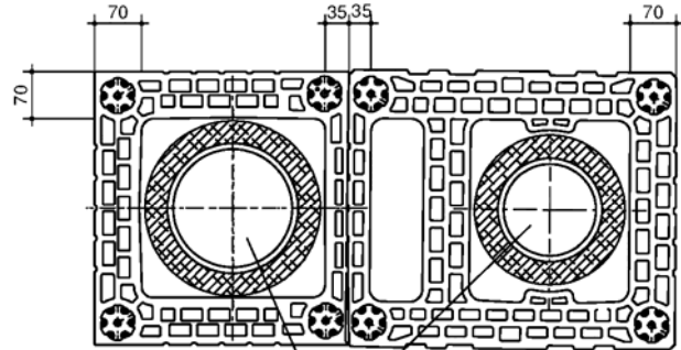
ZMS 42+ ZMS 42LR+ ERLUS Ek - Rohr
