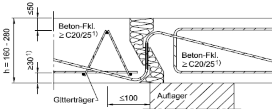
Abb. 41 Halfen-Iso-Element Typ HIT-VT mit Gitterträger
