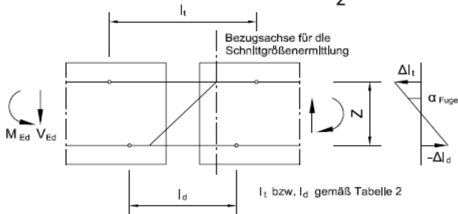
Abb. 31: Modell für die Ermittlung der Biegeverformung in der Fuge
