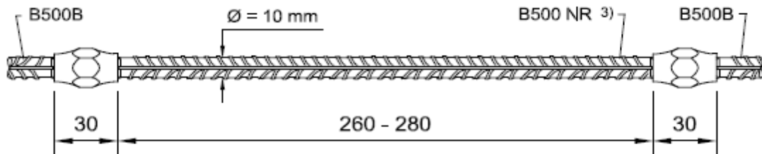
Abb. 13: Zugstab mit Verpressmuffe
