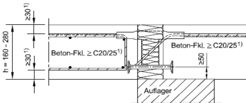
Abb. 16: Beispiel Halfen - Iso - Element Typ HIT-BX mit Aufhängebewehrung
