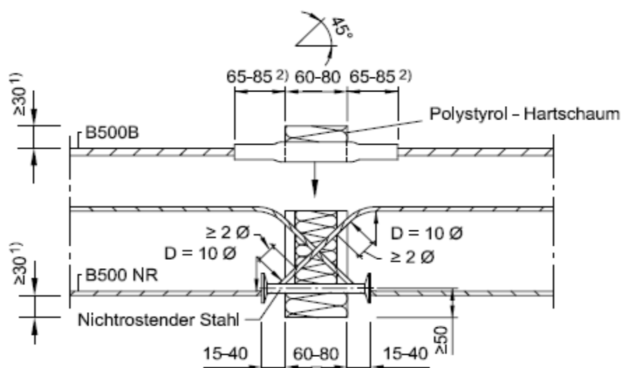
Abb. 17: Typ HIT-BF-±Q
