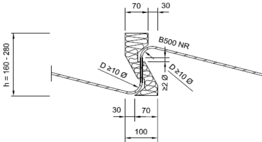
Abb. 40 Halfen-Iso-Element Typ HIT-VT
