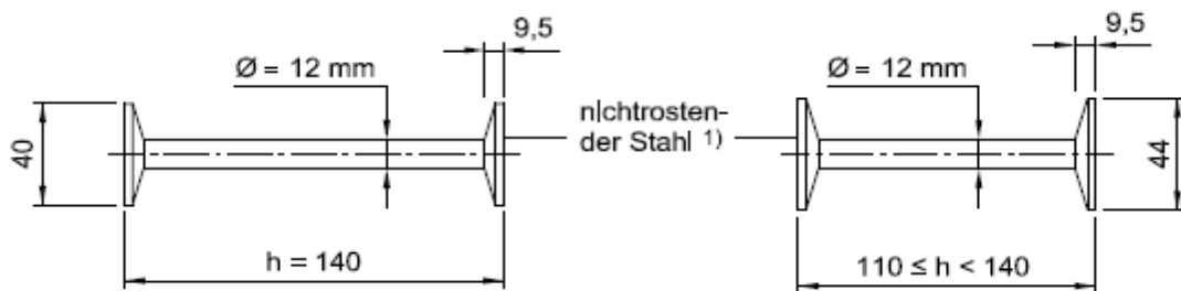
Abb. 17: Doppelkopf-Drucklager 2) aus nichtrostendem Stahl
