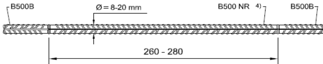
Abb. 15: Zugstab mit geschweißten Stößen
