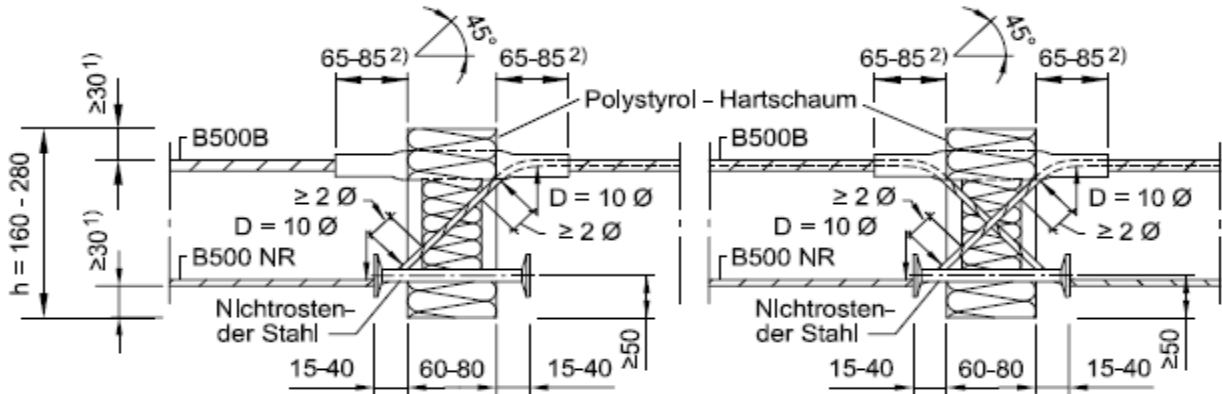
Abb. 13: Typ HIT-BX
