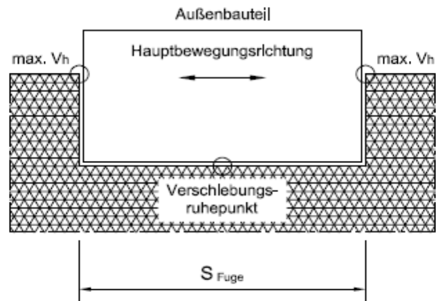
Abb. 30: Einbausituation mit Lagerung an gegenüberliegenden Rändern
