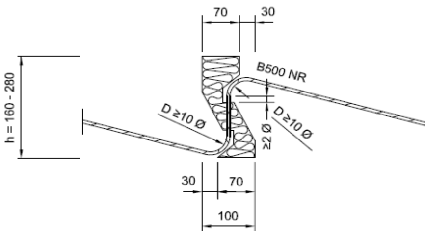
Abb. 22 Halfen-Iso-Element Typ HIT-VT
