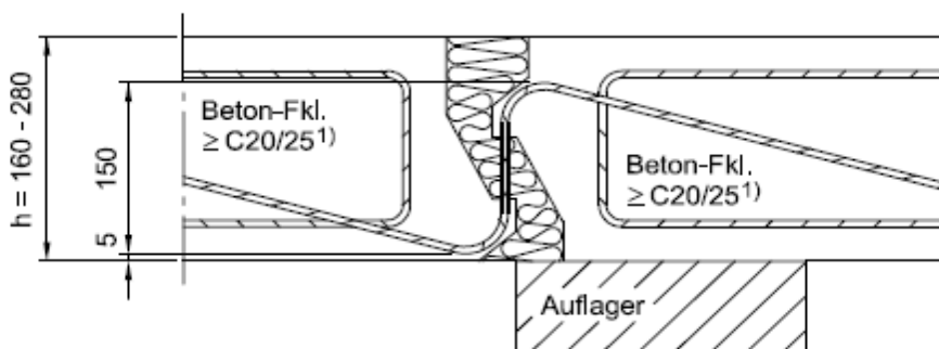
Abb. 23 Halfen-Iso-Element Typ HIT-VT mit Aufhängebewehrung
