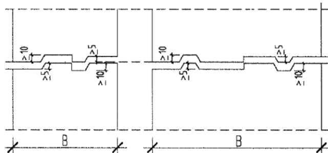
c. Stirnflächen mit wechselseitiger Nut und Feder
