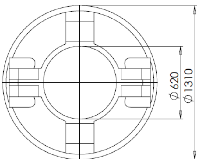
Draufsicht
